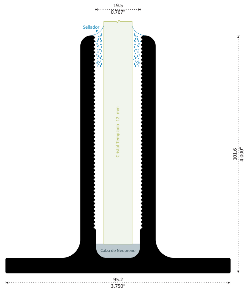
28009 ZOCLO BARANDAL Longitud: 6.10 m 28009-C 3.05 m
