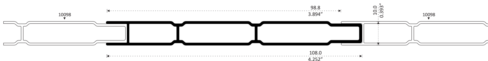
10098 PATENTE DUELA DOBLE VISTA 10 mm. Longitud 6.10 m 10098-5 5.00 m
