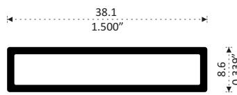
2503 RECTANGULAR 38.1 mm x 8.6 mm Longitud 6.10 m
