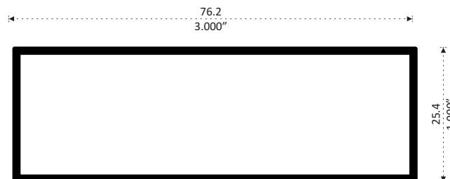
2516 RECTANGULAR 3" x 1" Longitud 6.10 m
