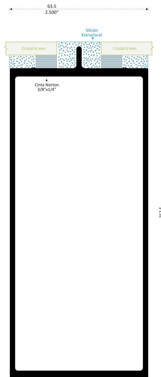
14739 BÁSICO TUBULAR INTEGRAL 6" X 2 1/2" Longitud 6.10 m
