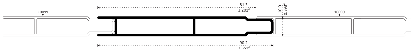
10099 PATENTE DUELA PARKET DOBLE VISTA Longitud : 6.10 m 10099-5 5.00 m
