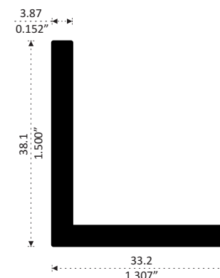
21311 Longitud 6.10 m Ángulo para Escuadras Puerta Batiente Comercial
