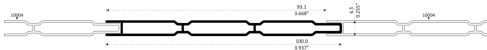
10004 PATENTE DUELA DOBLE VISTA 6.5 mm. Longitud 6.10 m 10004-5 5.00 m
