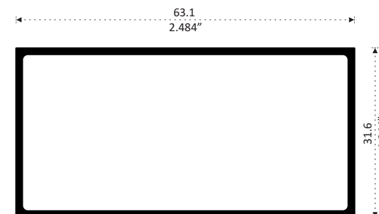
2513 RECTANGULAR 2 1/2" x 1 1/4" Longitud 6.10 m
