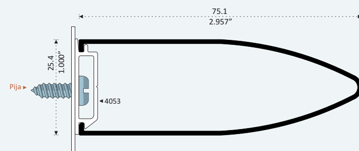
82516 ROMPE VISTA Longitud 6.10 m
