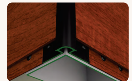
Colocación Duela Horizontal
