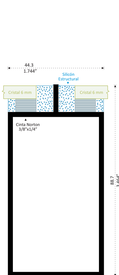
611003 BÁSICO TUBULAR INTEGRAL 3" X 1 3/4" Longitud 6.10 m
