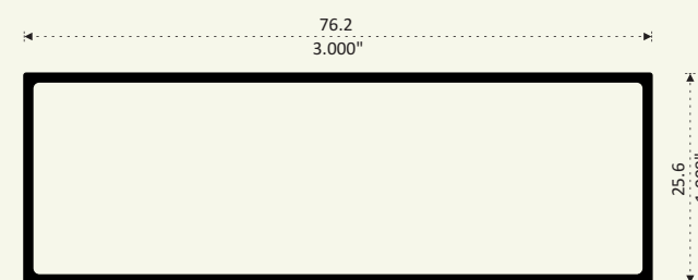
62516 RECTANGULAR LIGHT DE 3" X 1" Longitud 6.10 m
