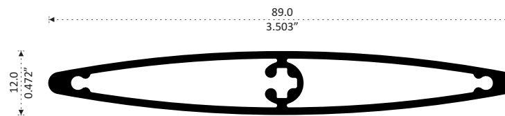
6054 ROMPE VISTA Longitud: 6.10 m
