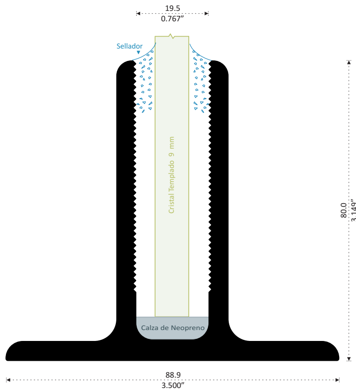
28008 ZOCLO BARANDAL Longitud: 6.10 m 28008-C 3.05 m
