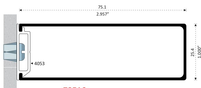
72516 ROMPE VISTA Longitud 6.10 m
