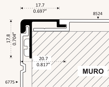
8522 ESQUINERO COMBINABLE Longitud 6.10 m
