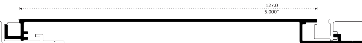
76617 DUELA LISA 5" Longitud: 6.10 m
