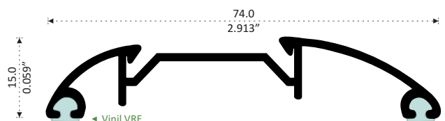
5019 REGLA DE CORTE Longitud: 5.80 m
