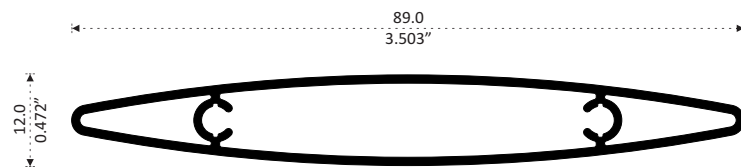
66054 PATENTE ROMPE VISTA Longitud: 6.10 m
