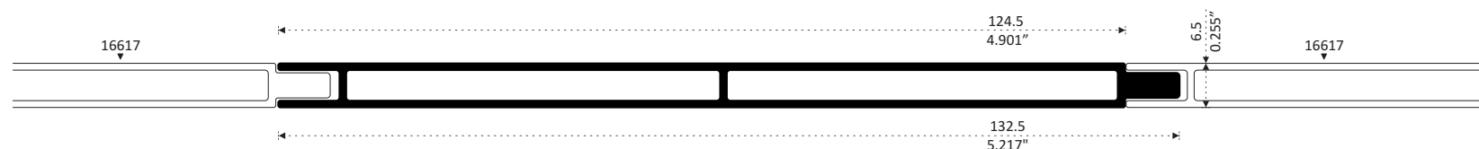
16617 PATENTE DUELA LISA DOBLE VISTA 5" Longitud : 6.10 m 16617-5 5.00 m
