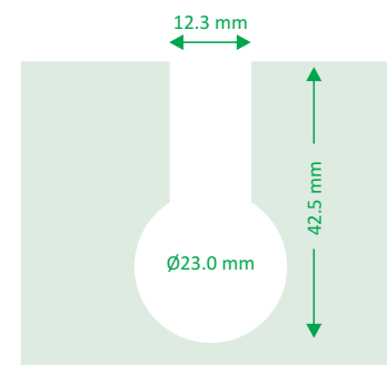
RESAQUE AL CRISTAL
