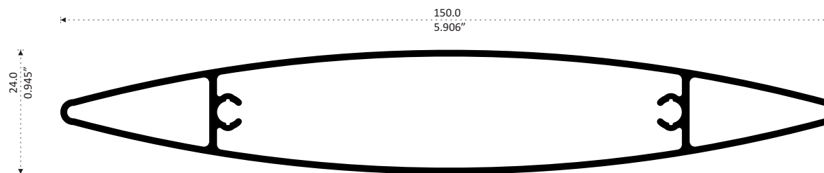
66055 ROMPE VISTA Longitud: 6.10 m
