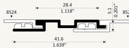
8520 PATENTE MOLDURA COMBINABLE Longitud 6.10 m
