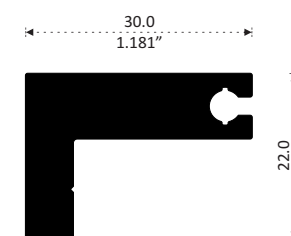
10201 ESCUADRA CON VENA Longitud 3.05 m
