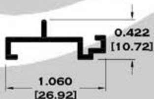
9966 ADAPTADOR MOSQUITERO
