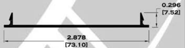
7316 TAPA LISA
