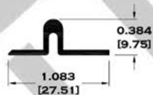
7818 RIEL ADAPTADOR
