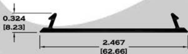
4130 TAPA BÁSICO
