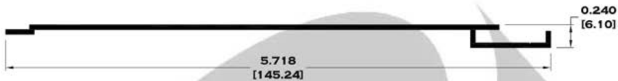
6617 DUELA LISA
