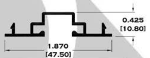
9085 TAPA BOLSA
