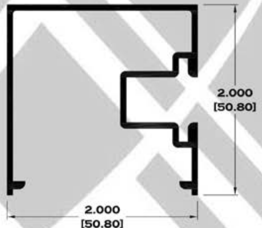
8586 ESQUINERO
