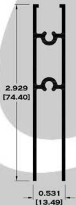
7825 ZOCLO PUERTA
