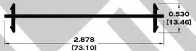
10266 MOLDURAUNIÓN
