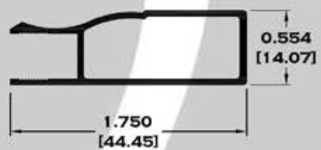
9756 MARCO SEMILUJO
