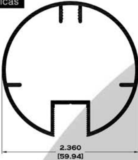
23896 PASAMANOS REDONDO 2"
