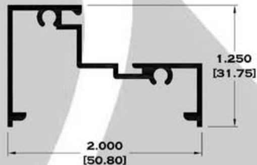
9084 ESCALONADO
