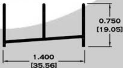
11388 RIEL INFERIOR
