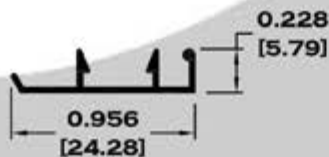
7333 MOSQUITERO
