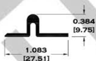
7818 RIEL ADAPTADOR
