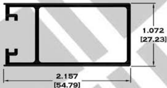
9236 CERCO CHAPA
