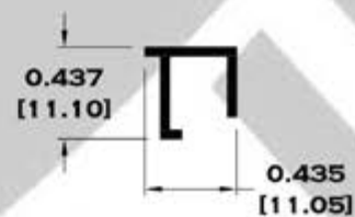
7014 JUNQUILLO
