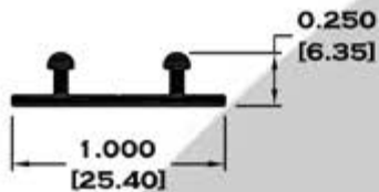
3316 RIEL VITRINA
