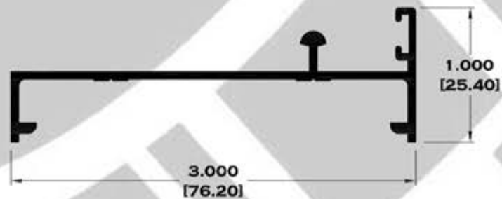
9957 RIEL
