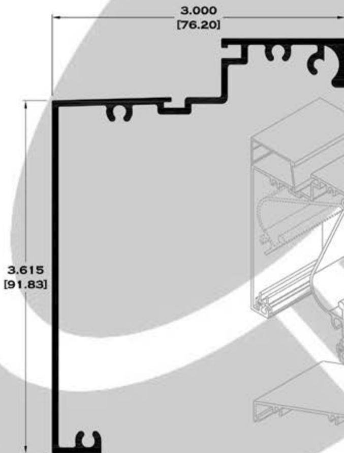
10465 CABEZAL ESCALONADO
