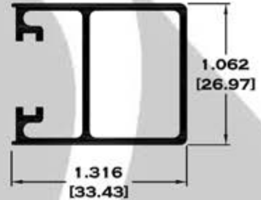
7843 CERCO VENTANA
