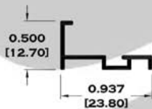
7013 PORTAVIDRIO
