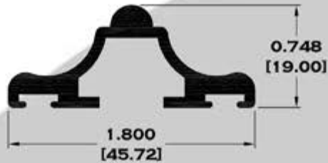
033 MOLDURA
