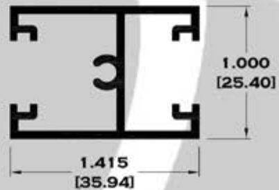
9082 INTERMEDIO
