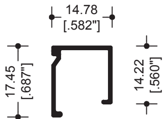
36370 JUNQUILLO
