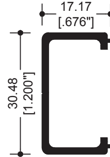
9965 CERCO FIJO
