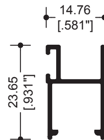
15312 CERCO
