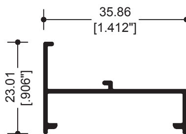
15313 ESCALONADO PRODUCCIÓN
