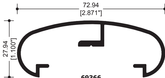
69366 PASAMANOS 3"
