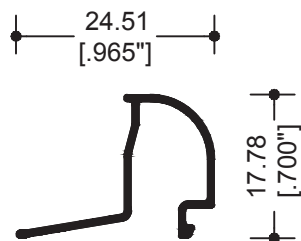
69887 JUNQUILLO CONCAVO DOBLE
