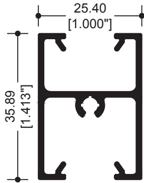
69082 INTERMEDIO
