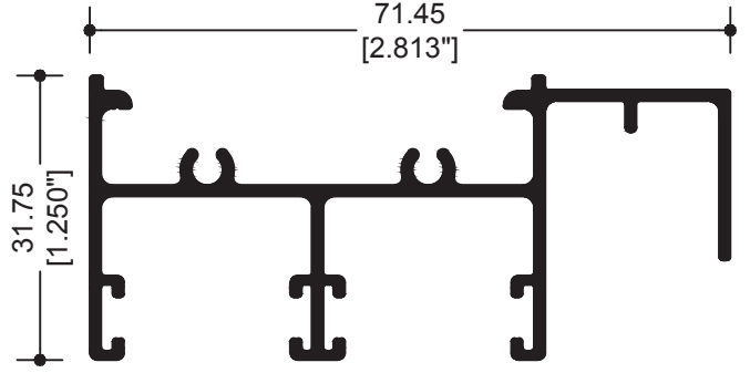
27819 CABEZAL MOS. CORREDIZO
