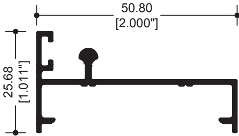
14286 RIEL
