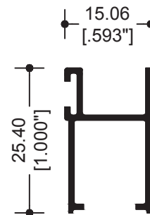
11836 CERCO
