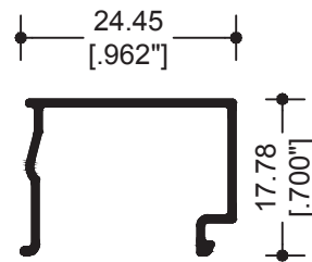
69890 JUNQUILLO CUADRADO SENCILLO
