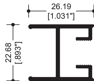
7107 CERCO FIJO
