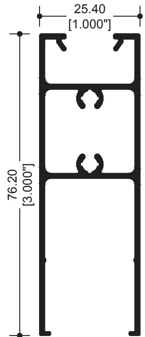
67842 ZOCCO
