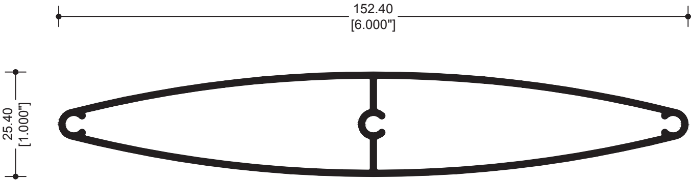
67362 CELOSÍA 6"
