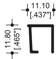
15314 JUNQUILLO PRODUCCIÓN
