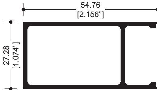
9964 CERCO PUERTA DOBLE VIDRIO
