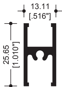
11203 INTERMEDIO PARA CUADRÍCULA
