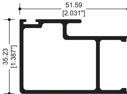
9963 TRASLAPE PUERTA DOBLE VIDRIO
