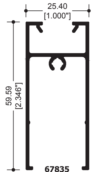
67835 ZOCLO VENTANA
