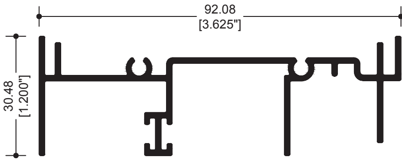
7109 CABEZAL CONTRAMARCO CORREDIZA
