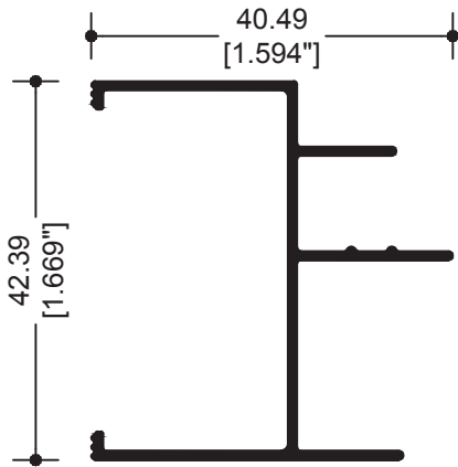
10570 JAMBA
