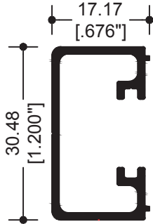
28681 ADAPTADOR FIJO
