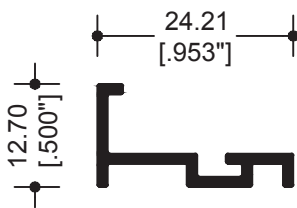
67013 BASE
