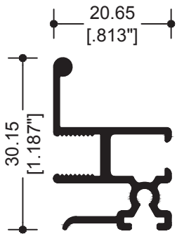
10571 CERCO MÓVIL
