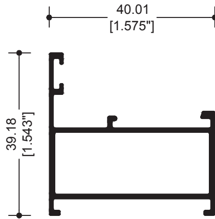
69877 MARCO VENTANA
