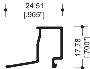
69888 JUNQUILLO CUADRADO DOBLE
