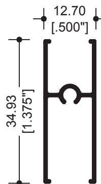
15311 CABEZAL Y ZOCLO
