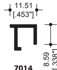
7014 JUNQUILLO
