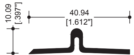
7828 ADAPTADOR XX
