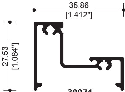
39074 ESCALONADO
