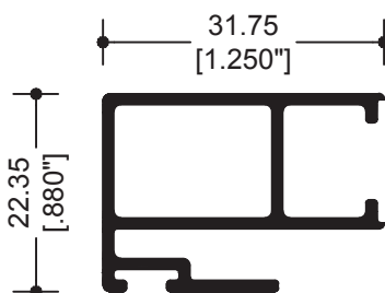
39954 TRASLAPE VENTANA
