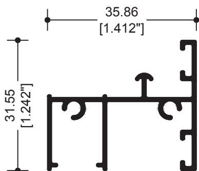
63862 INTERMEDIO PRODUCCIÓN
