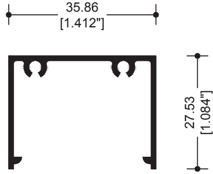
29076 BOLSA LISA
