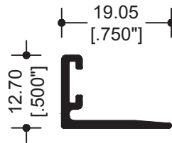
11032 BATIENTE
