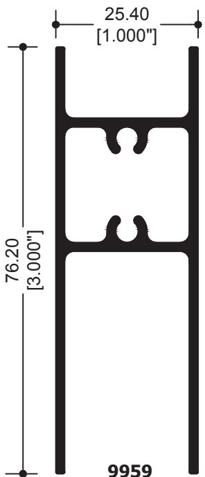
9959 ZOCLO PUERTA VIDRIO DOBLE
