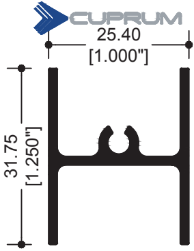
9958 CABEZAL DUO VENT
