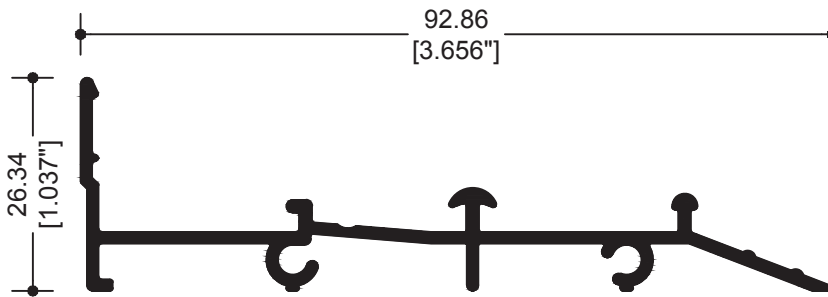
7110 RIEL CONTRAMARCO CORREDIZO
