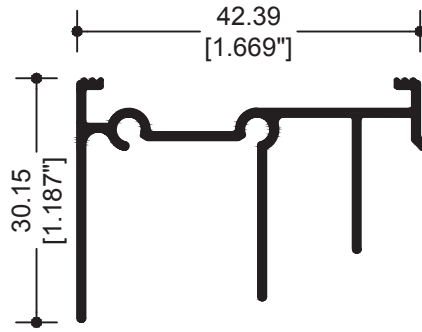
10568 CABEZAL
