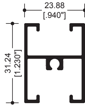
69768 INTERMEDIO
