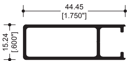
67821 CERCO PUERTA
