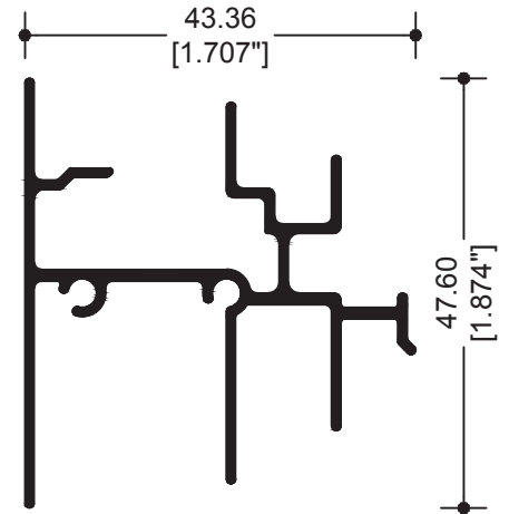
12797 RIEL Y CABEZAL
