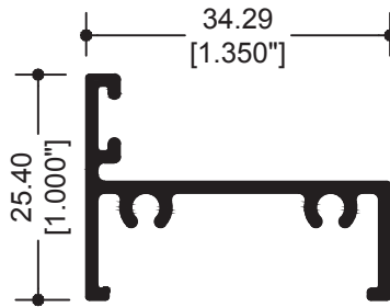
33087 MARCO PARA PUERTA
