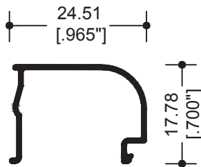
69891 JUNQUILLO CONCAVO SENCILLO
