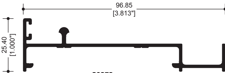
39272 RIEL PARA MOS. EXT. CORREDIZO
