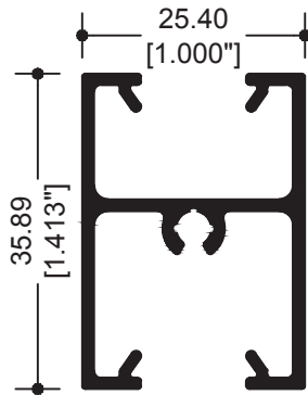
69082 INTERMEDIO
