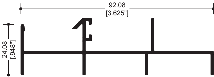
27111 JAMBA PARA CORREDIZA
