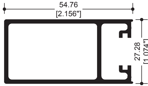
9236 CERCO CHAPA
