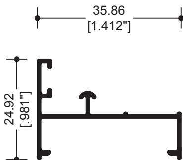
15310 RIEL
