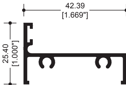
68550 MARCO PARA PUERTA
