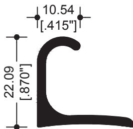
4154 JALADERA
