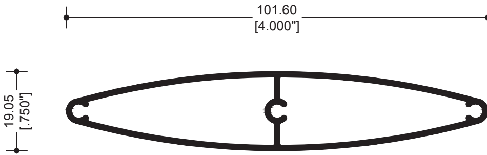
67363 CELOSÍA
