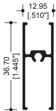
11837 CABEZAL Y ZOCLO
