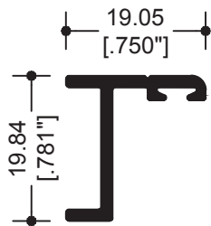
4127 BATIENTE
