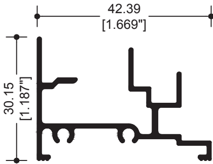
20569 RIEL
