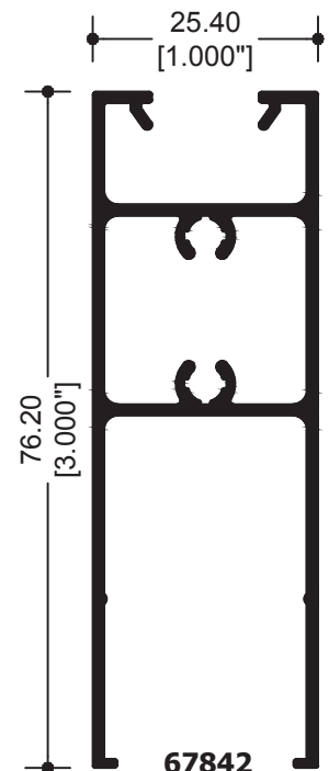
67842 ZOCLO PUERTA
