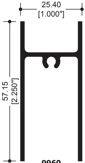
9960 ZOCLO VENTANA VIDRIO DOBLE
