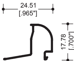
69887 JUNQUILLO CONCAVO DOBLE
