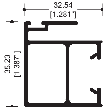
67844 CERCO TRASLAPE VENTANA
