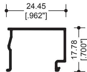
69890 JUNQUILLO CUADRADO SENCILLO
