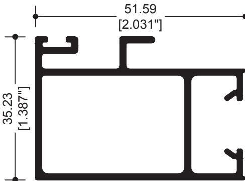
67848 TRASLAPE PUERTA
