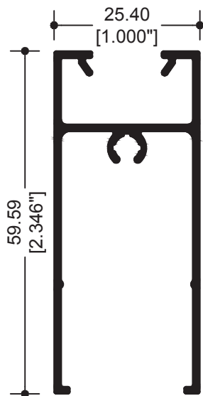
67835 ZOCCO
