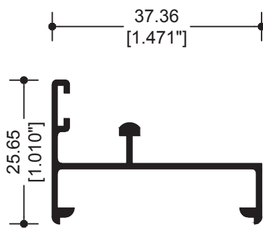
11838 RIEL
