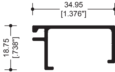
28939 JUNQUILLO
