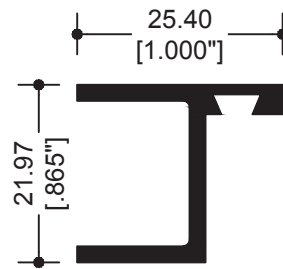
7102 BATIENTE
