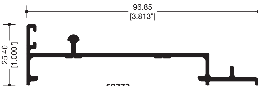
69272 RIEL PARA MOS. EXT. CORREDIZO
