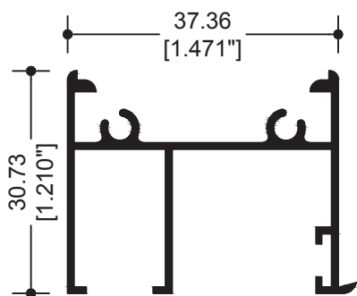
11835 JAMBA Y CABEZAL
