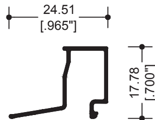
69888 JUNQUILLO CUADRADO DOBLE
