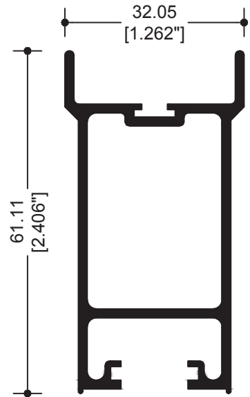
67850 CERCO OXXO
