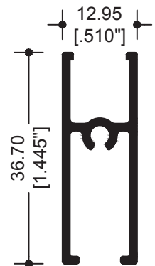
9956 CABEZAL Y ZOCLO
