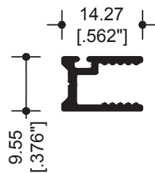
10574 CERCO FIJO
