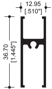
11044 CABEZAL Y ZOCLO
