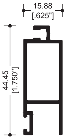
66534 CERCO MOSQUITERO
