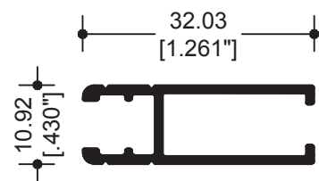
53358 ZAPATA
